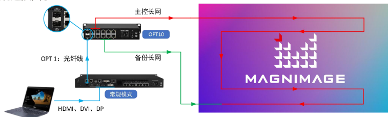
光口复制连接图示:
