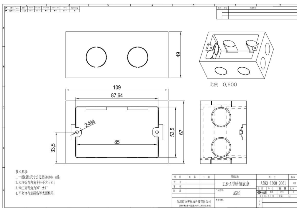
电源盒（电源选配）尺寸图
