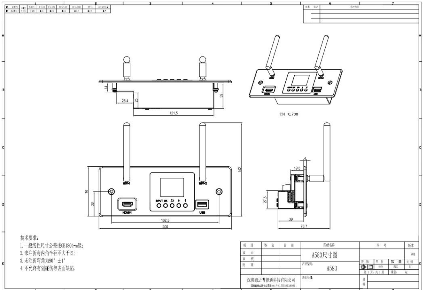
LED-F486 尺寸图
