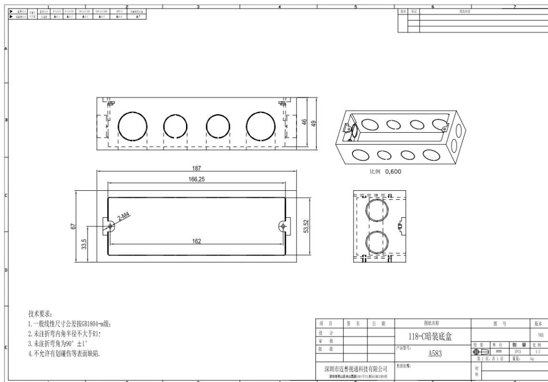
86 盒尺寸图
